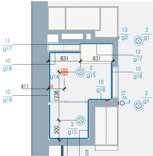
Фрагмент 1 плана освітлення (розміщення підсвітки під тумбою умивальника)
