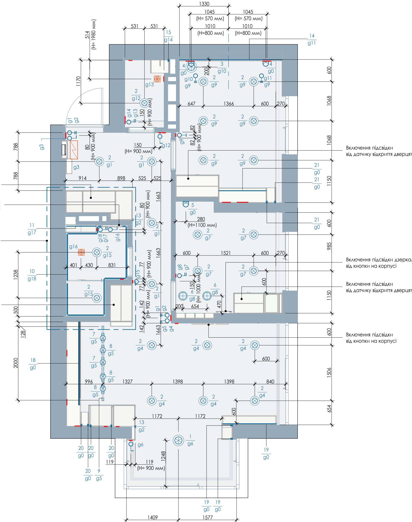
Фрагмент 1 плана освітлення (розміщення підсвітки під тумбою умивальника)
